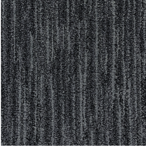
Magnetite
