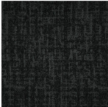
Magnetite
